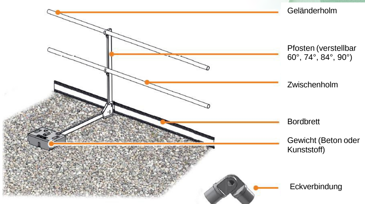
Bild 1: Seitenschutzsystem, Typ: TigaRAIL
