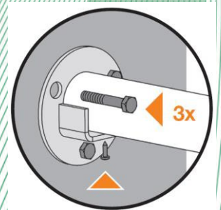
Bild 8: Holmhalter
