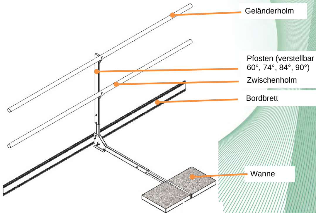
Bild 16: Seitenschutzsystem, Typ: TigaraIL PLUS WANNE
