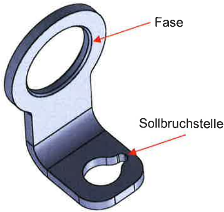
Bild 4: Anschlagpunkt, Typ: TS-Lasche (TS-011) (mit Sollbruchstelle, mit Fasen (1 x 45°))
