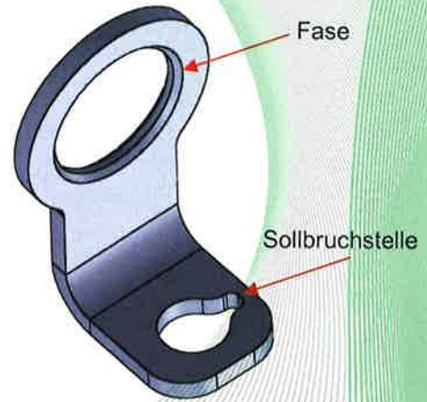
Bild 5: Anschlagpunkt, Typ: TS-Lasche (TS-011) (mit Sollbruchstelle, mit Fasen (1,5 x 45°))
