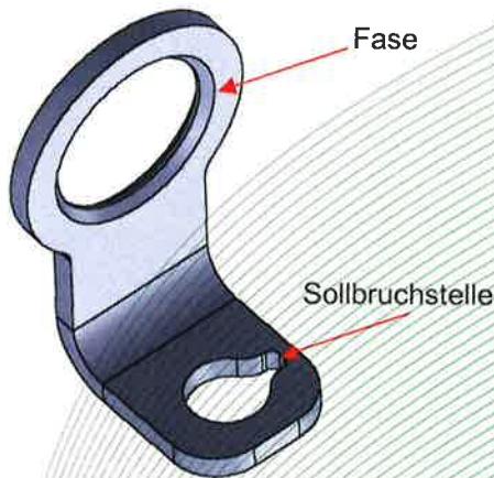
Bild 6: Anschlagpunkt, Typ: TS-Lasche (TS-011) (mit Sollbruchstelle, mit Fasen (2 x 45°))
