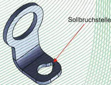
Bild 2: Anschlagpunkt, Typ: TS-Lasche (TS-106_V20) (mit Sollbruchstelle, ohne Fase)
